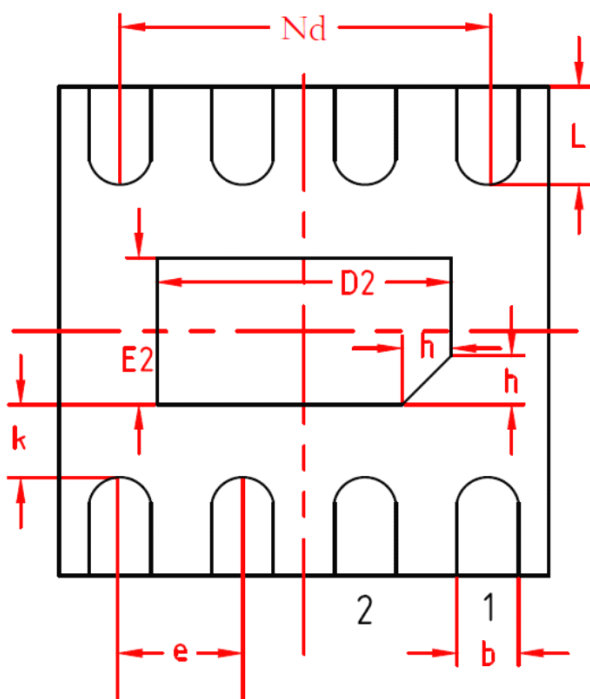
BOTTOM VIEW(背视图)
